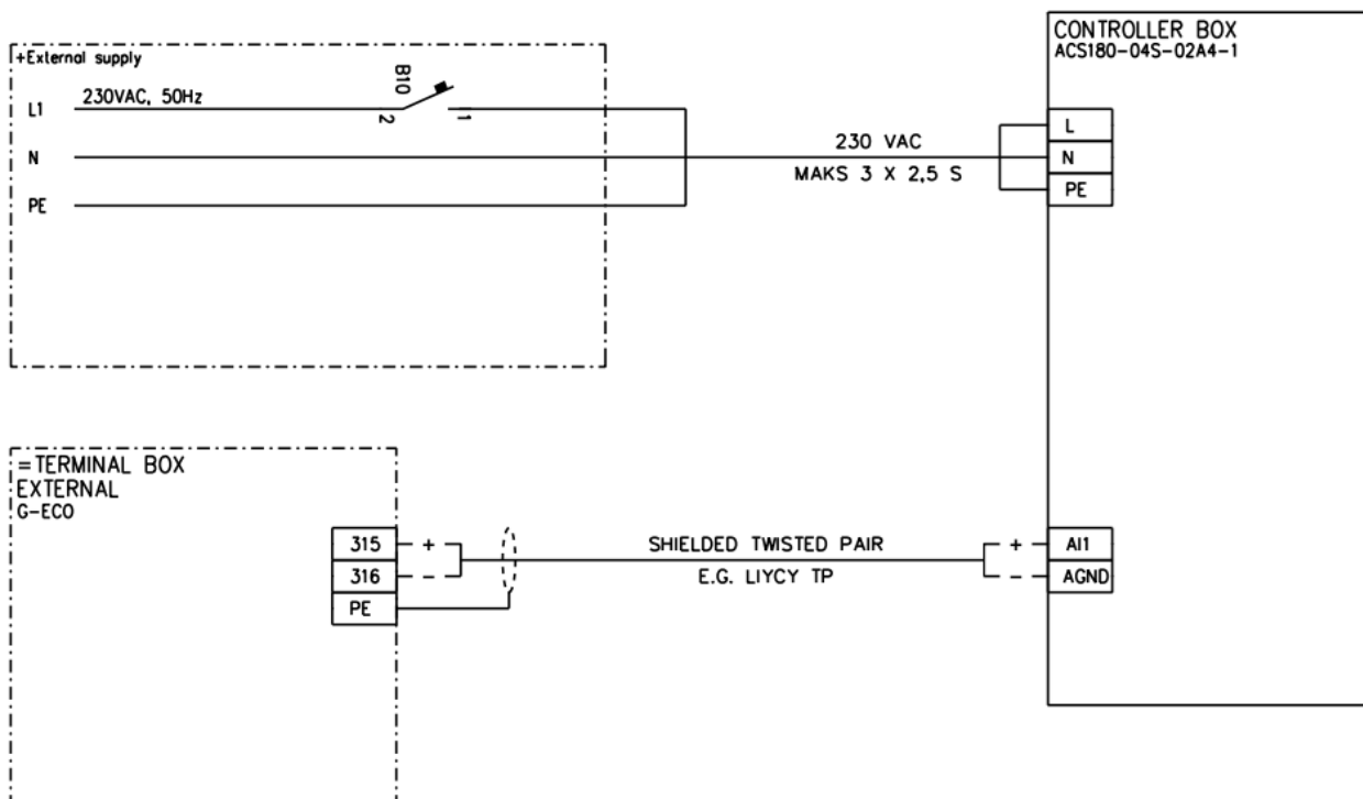
Bild 6.2 Kopplingsschema för styrdon till frånluftsfläkt
