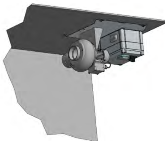
Bild 5.6 Vägghmontering
