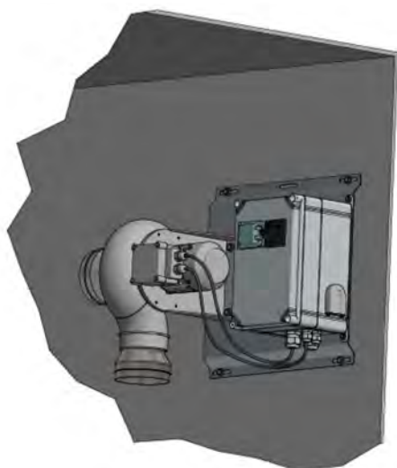
Bild 5.5 – Vägghmontering
