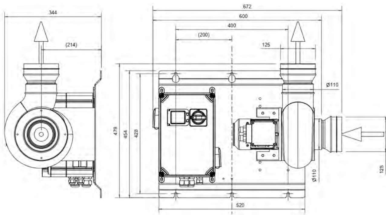
Bild 5.1 GebEF1 installationsmått
