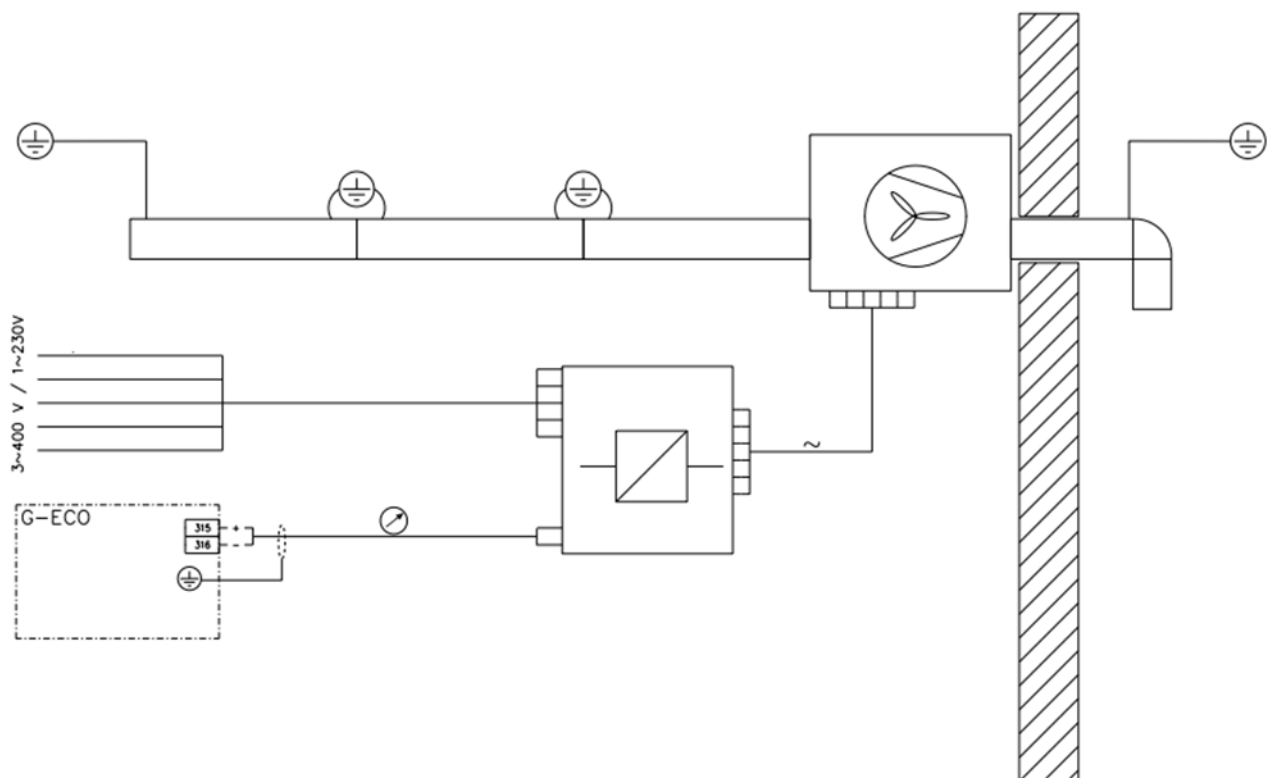
Bild 6.1 Anslutningsschema för frånluftsfläkten
