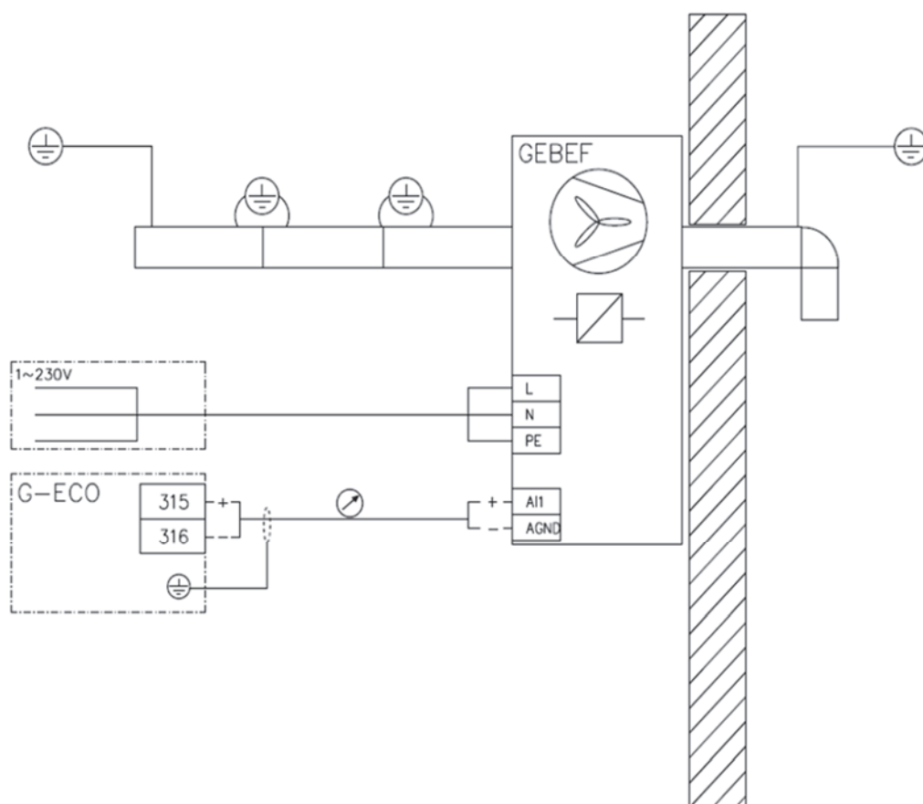
Bild 6.1 Anslutningsschema för frånluftfläkten
