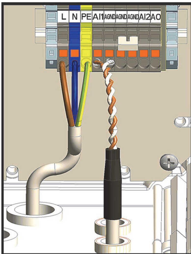
Bild 6.2 Styrdonets inkoppling
