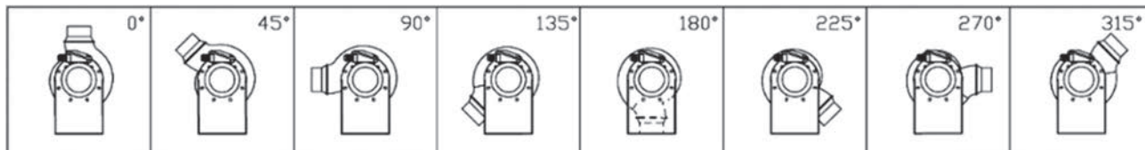
Bild 5.7 – Alternativa monteringslägen för fläkten
